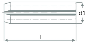
Maße und Bezeichnung größer 8 mm Nenndurchmesser
