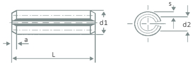
Maße und Bezeichnung bis 8 mm Nenndurchmesser
